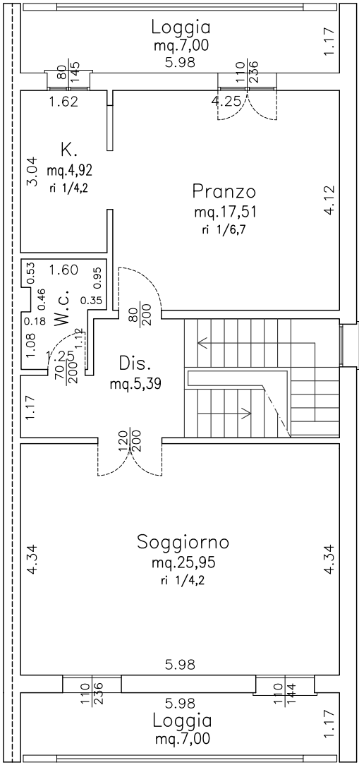
PIANO PRIMO Scala 1:100
