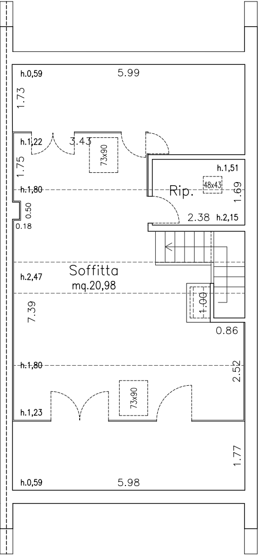
PIANO TERZO Scala 1:100
